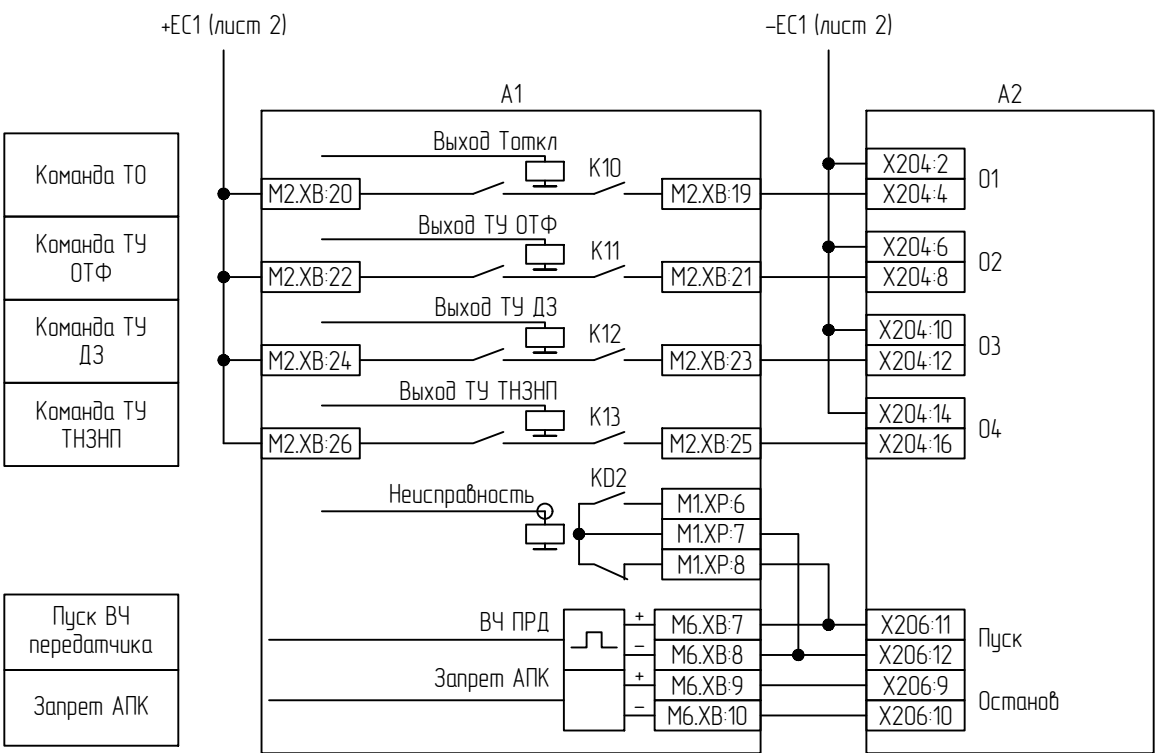
Цепи оперативного тока
