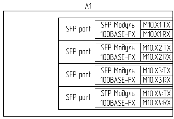
Цепи портов связи терминала
