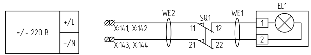
Цепи освещения шкафа
