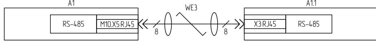
Цепи связи терминала с ИЧМ
